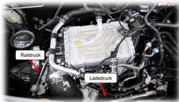
EA 288 ANALOGER LADEDRUCK 64 MHz
